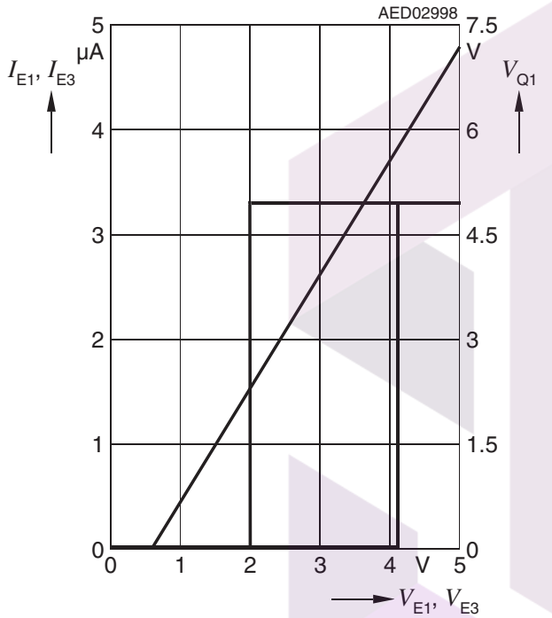
Enable Currents I_{E1} , I_{E3} and Output Voltage V_{Q1} versus Enable Voltages V_{E1} , V_{E3}
